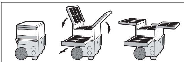
Ouverture des panneaux solaires
